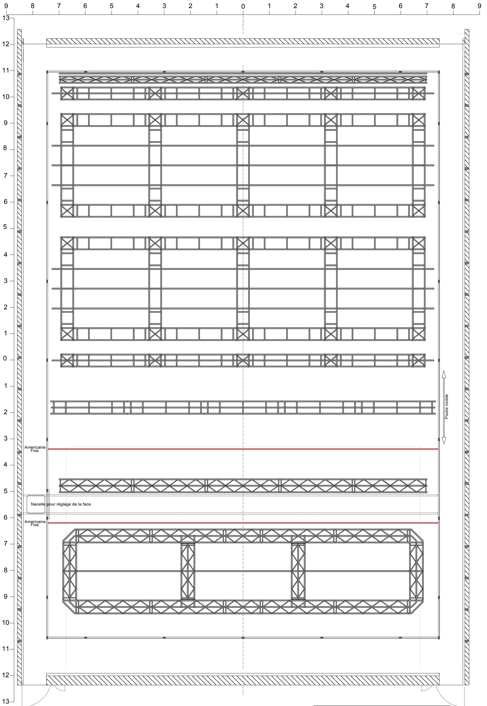
PAVILLON DE LA DANSE GENEVE PLATEAU PLAN DE MASSE PASSERELLES + TRUSS Ech 1/75 10/07/23
