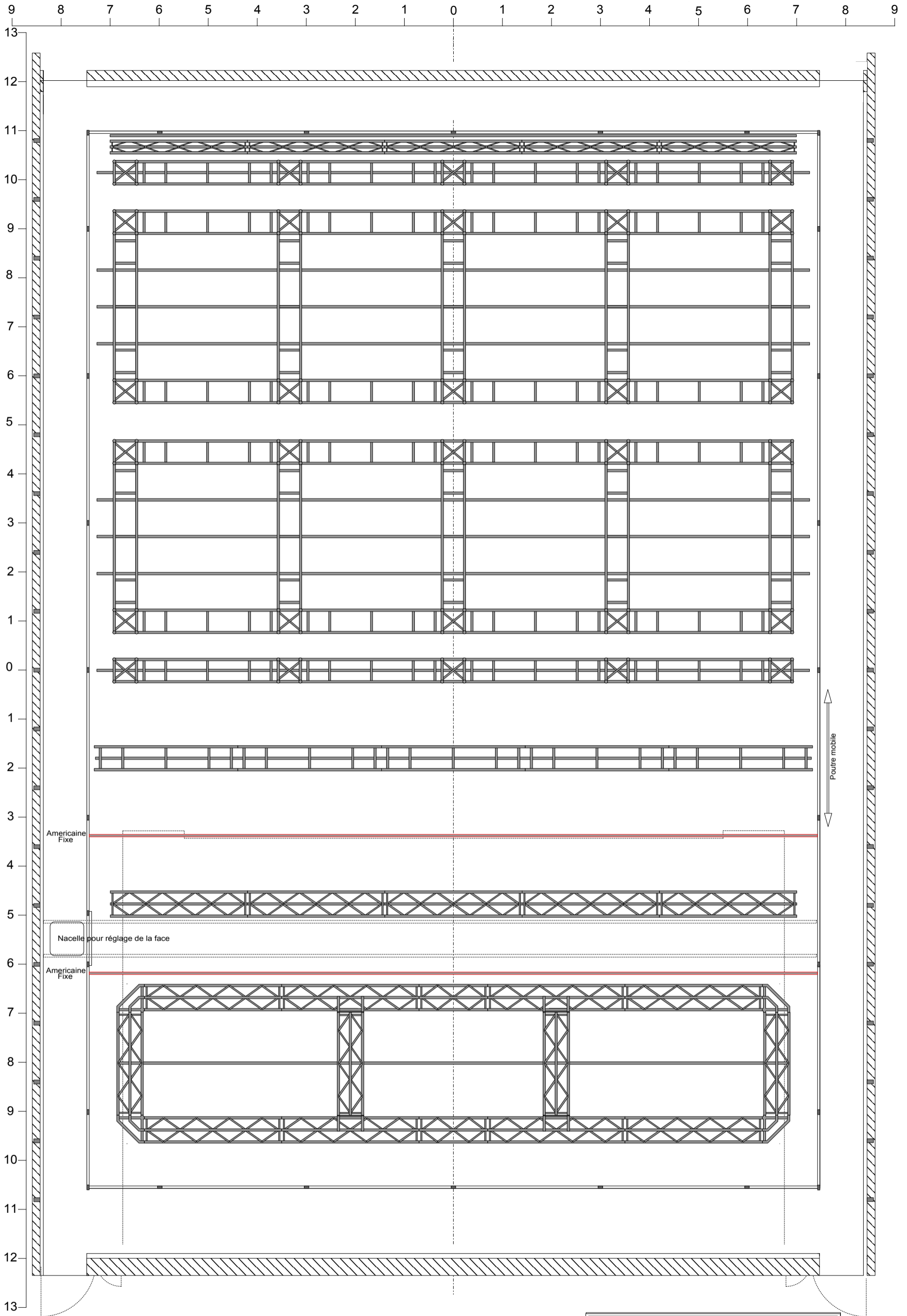
PAVILLON DE LA DANSE GENEVE PLATEAU PLAN DE MASSE PASSERELLES + TRUSS Ech 1/75 08/12/23
